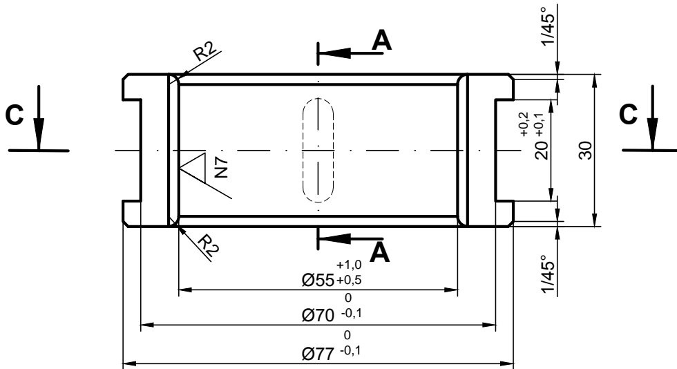
PRESEK "B-B"
