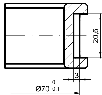
PRESEK "A-A"
